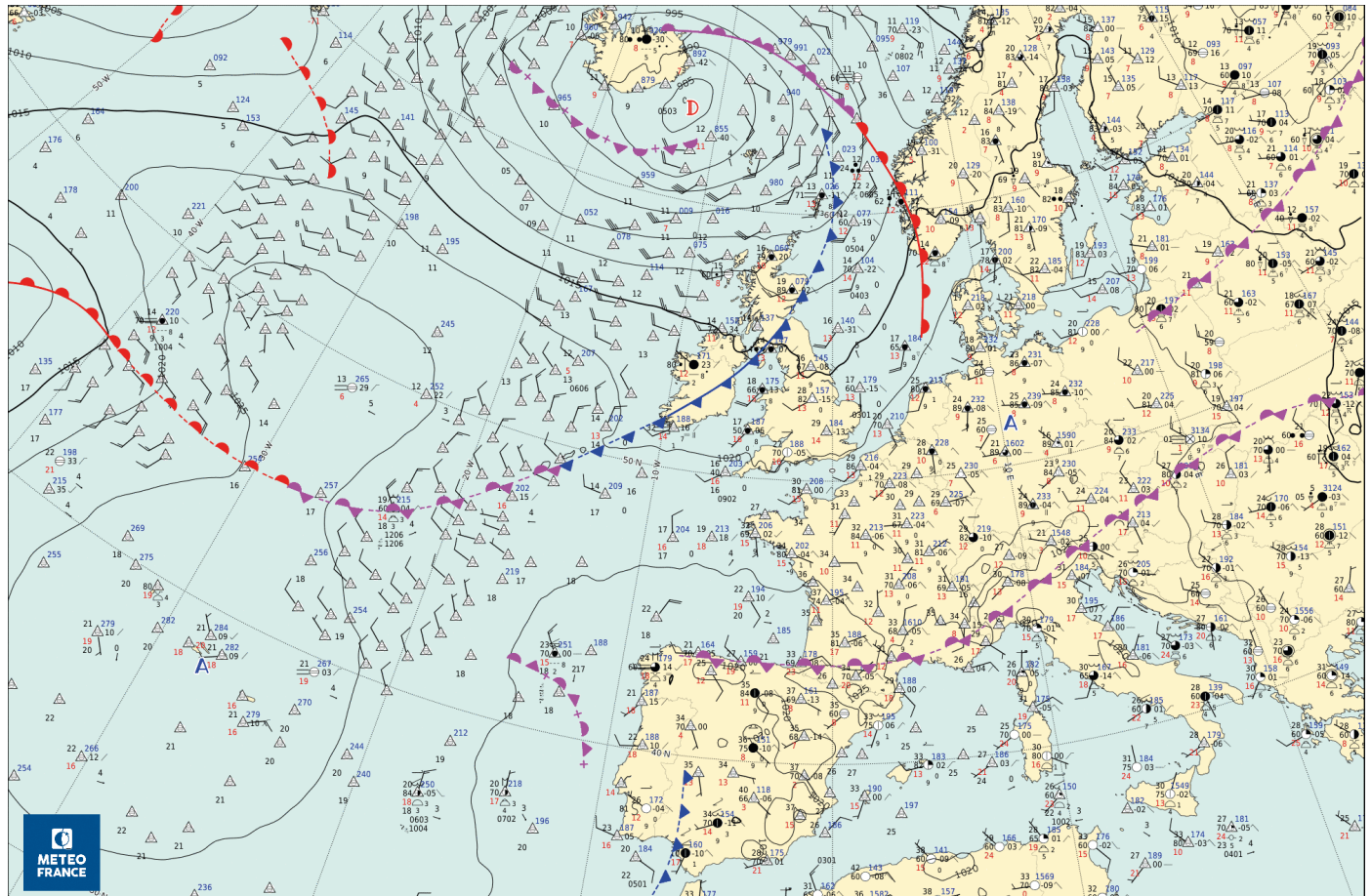
ANALYSE EN SURFACE du vendredi 17/06/2022 - 12 UTC
