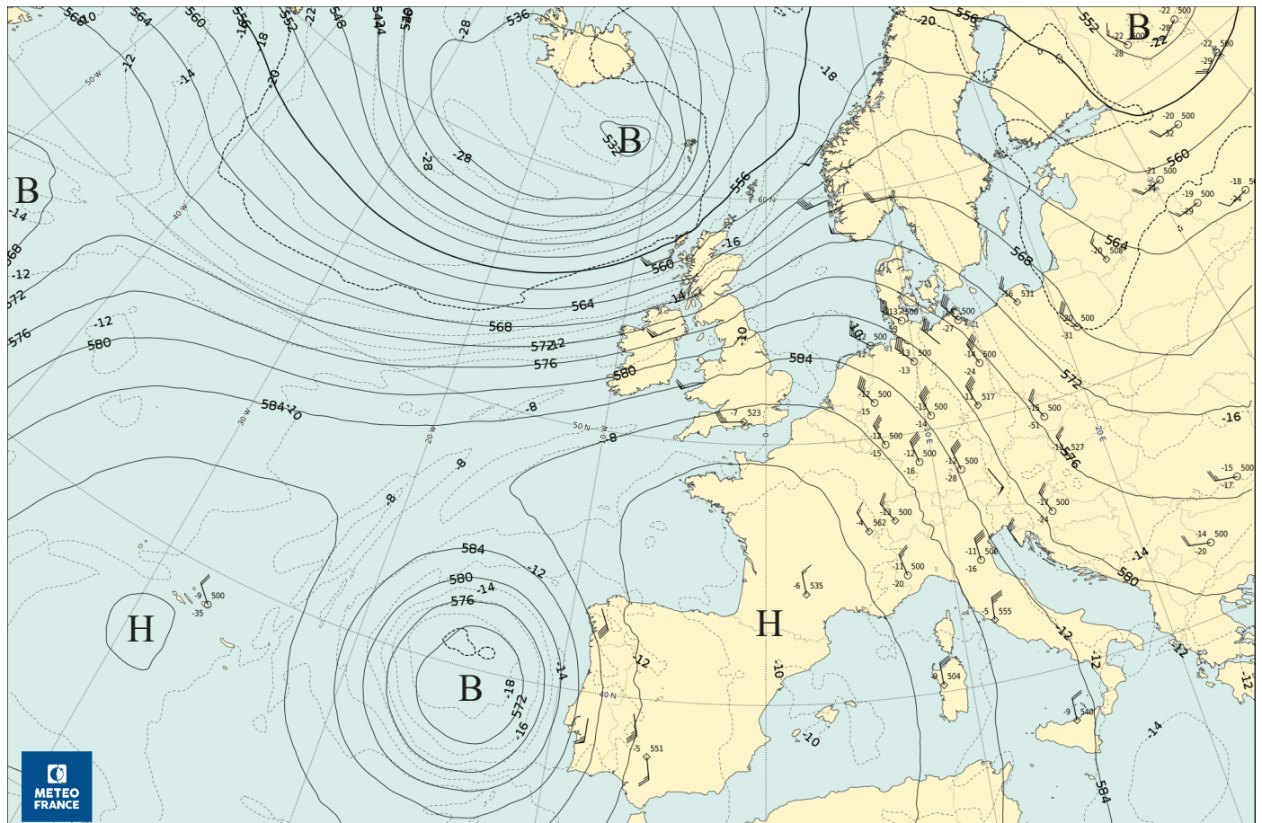
ANALYSE A 500hPa du vendredi 17/06/2022 - 12 UTC
