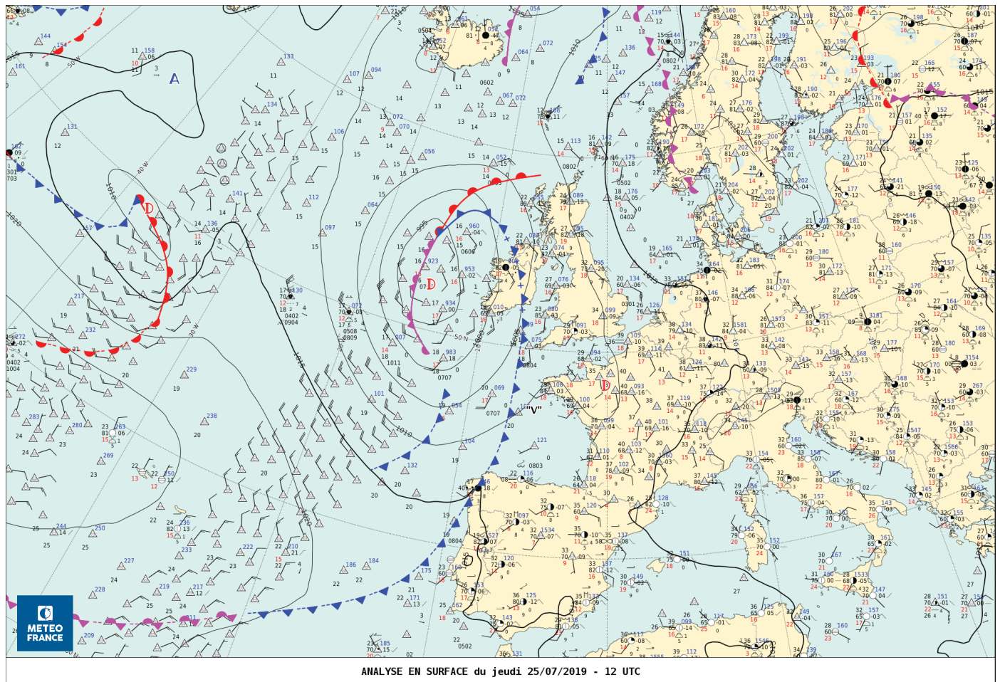
ANALYSE EN SURFACE du jeudi 25/07/2019 - 12 UTC
