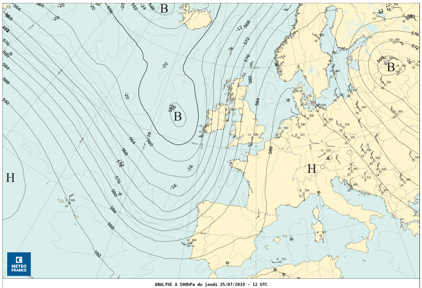
ANALYSE A 500hPa du jeudi 25/07/2019 - 12 UTC
