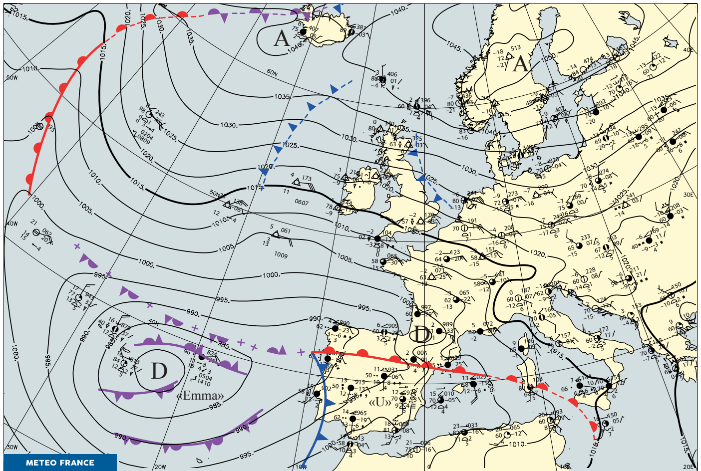
ANALYSE EN SURFACE DU MER 28/02/18 12UTC
