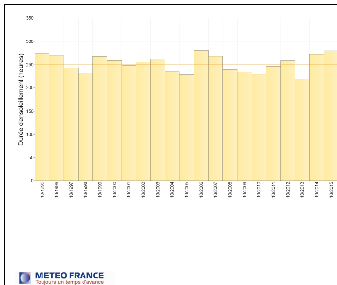
Cumul mensuel des durées d'ensoleillement à Pamandzi pour les mois d'octobre de 1995 à 2015
