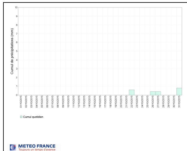
Cumul quotidien des précipitations à Pamandzi du 1er octobre 2015 au 31 octobre 2015
