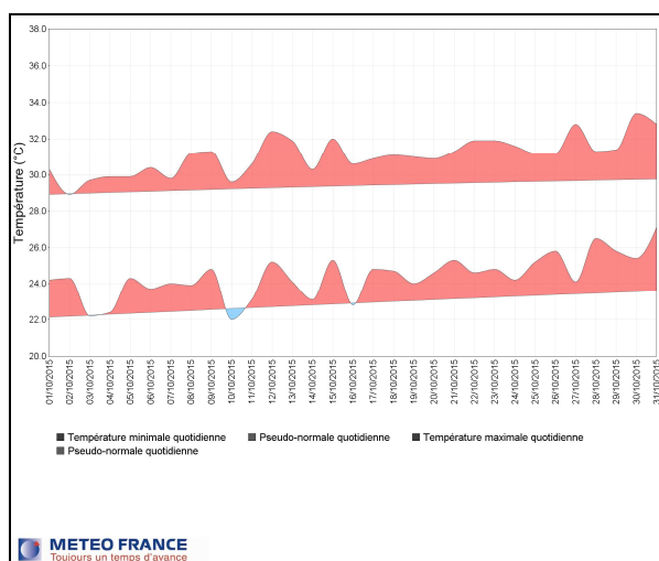
Températures minimales et maximales quotidiennes à Pamandzi du 1 er au 31 octobre 2015.
