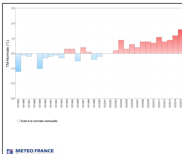
Ecart à la normale mensuelle de référence 1981-2010 de la température moyenne à Pamandzi pour octobre.
